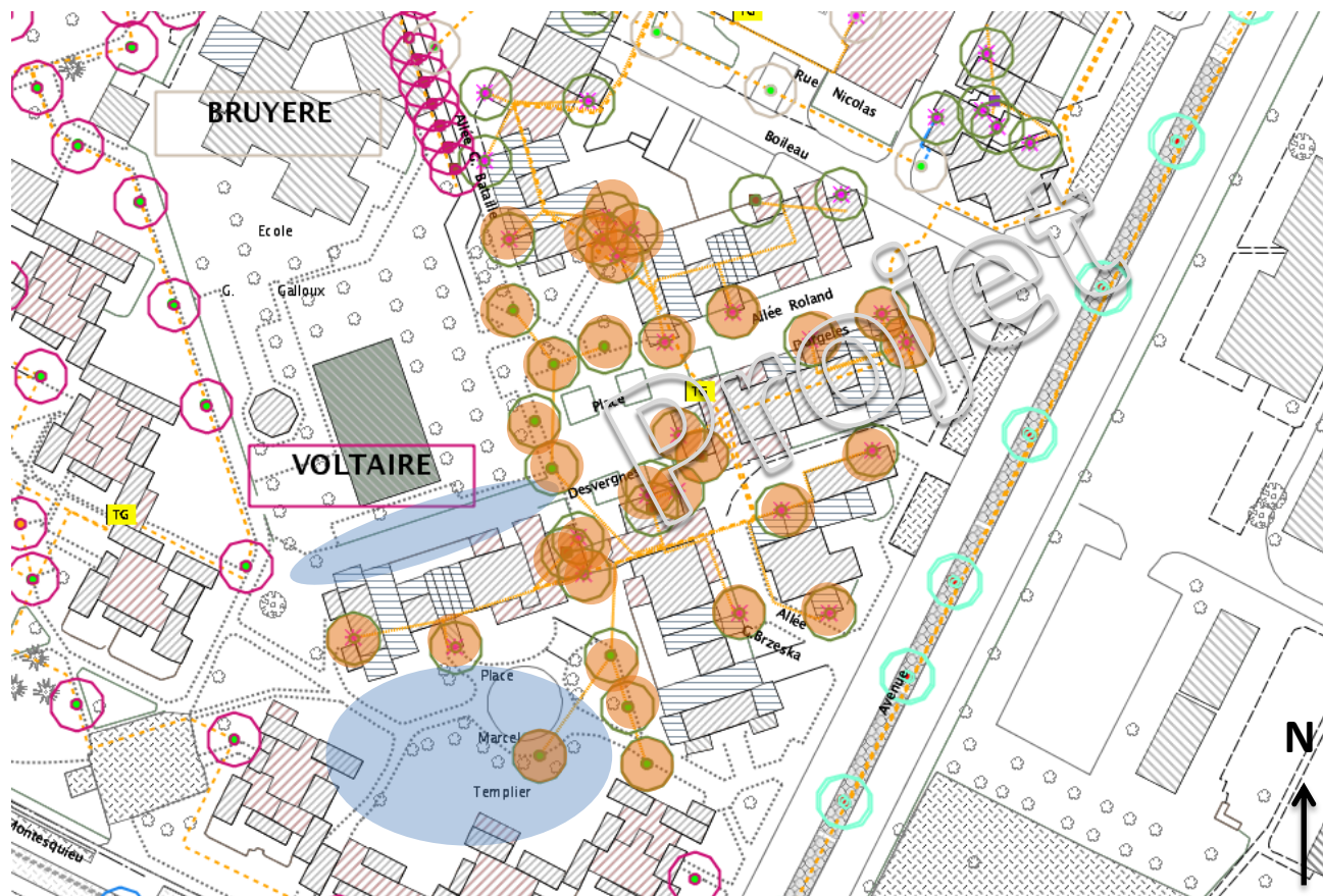
Plan de l'éclairage existant actuellement sur site
