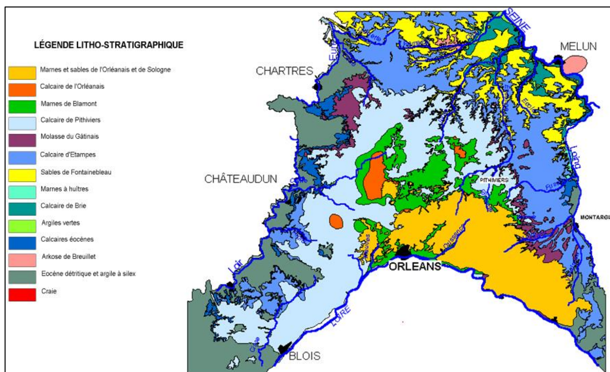
Litho-stratigraphie du complexe aquifère des Calcaires de Beauce (Rapport du BRGM R 40571)
